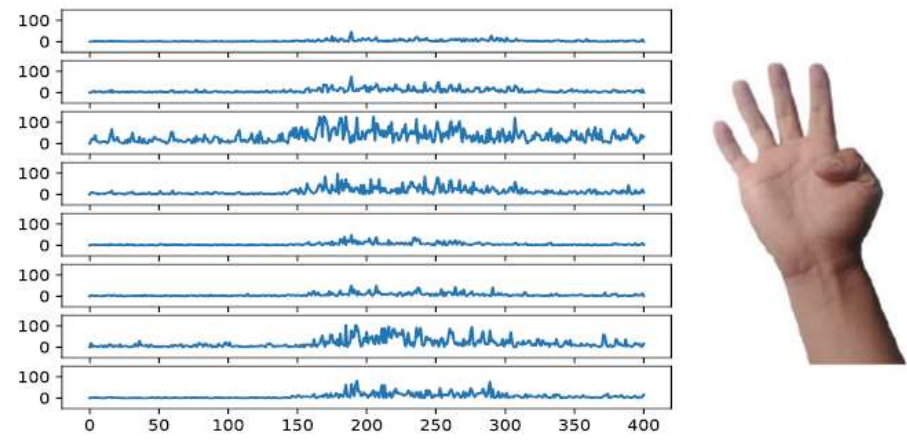
Figura 4. Señales EMG's para un arreglo de 8 electrodos.
